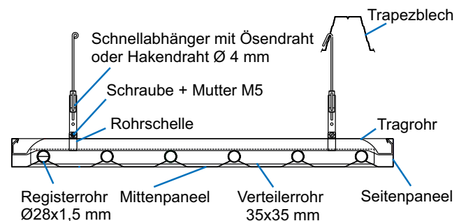
Querschnitt DSP Typ HB-150 ECO EVO
